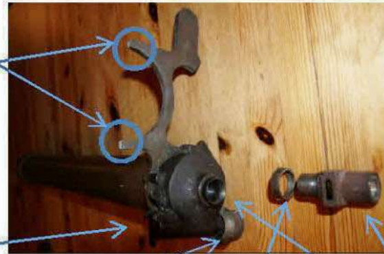
Bruchstellen an der Halterung
